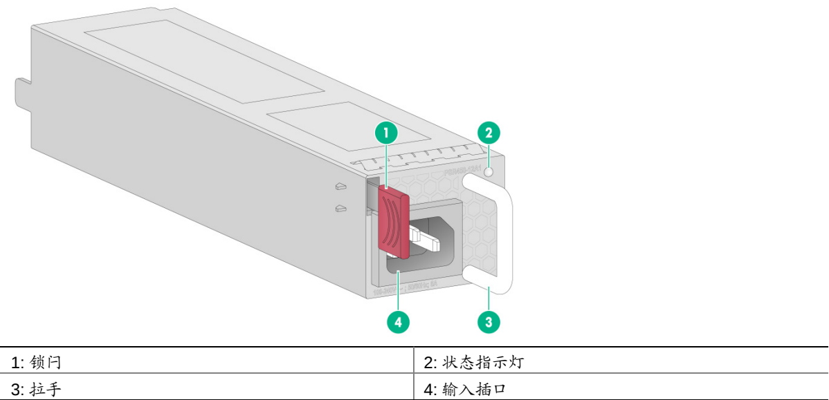
图1-6 交流电源模块正视图
