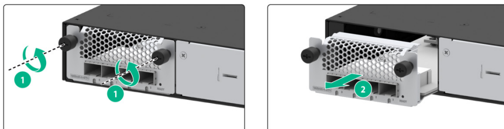
图4-2 拆卸接口模块
