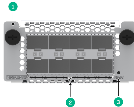
图1-4 NS-HPIM-GP8B-Z 接口模块正视图
