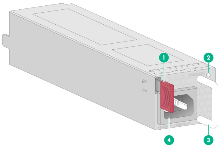
图1-5 交流电源模块正视图
