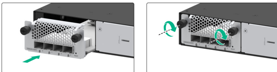
图2-10 安装接口模块
