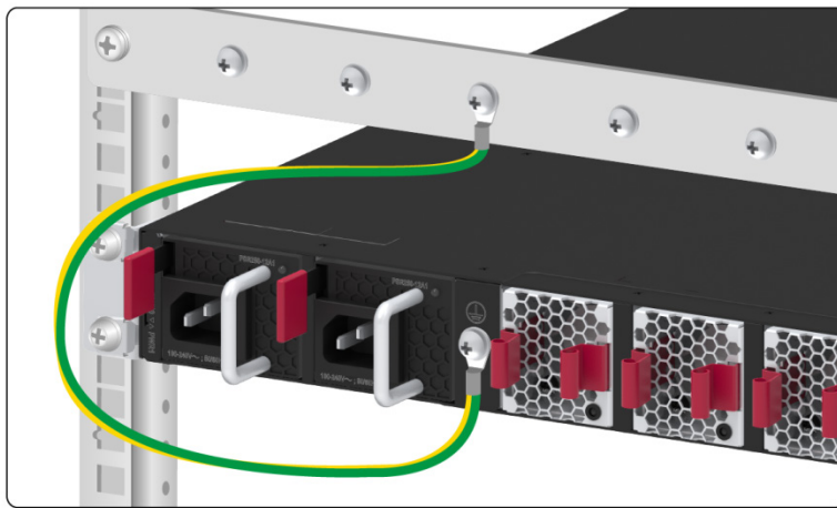
图2-7 连接到机柜接地
