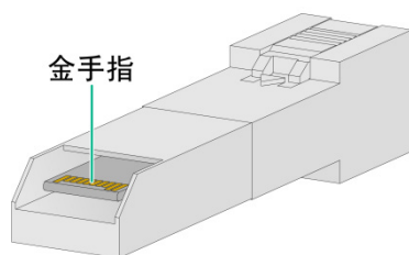
图4-4 光模块金手指
