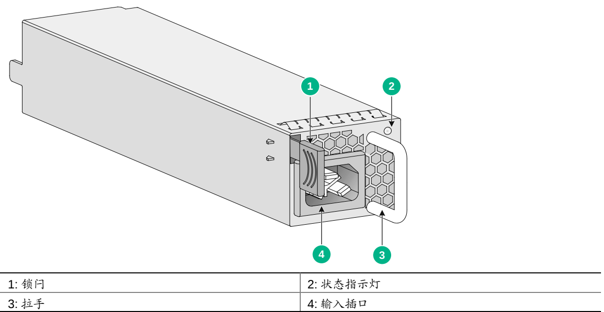
图1-8 高压直流电源模块外观
