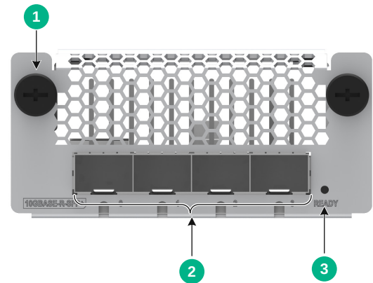
图1-3 NS-HPIM-TG4B-Z 接口模块正视图
