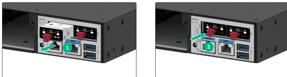
图2-11 安装硬盘
