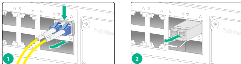
图4-5 拆卸光接口模块示意图
