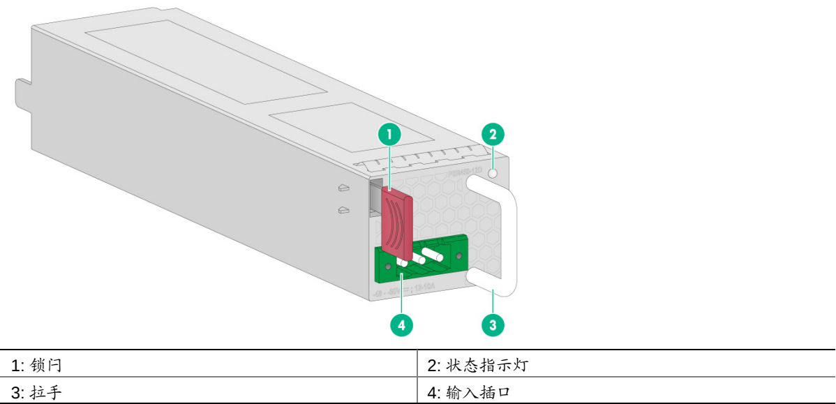
图1-7 直流电源模块正视图
