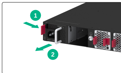
图4-1 拆卸电源模块
