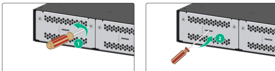
图2-9 拆卸假面板
